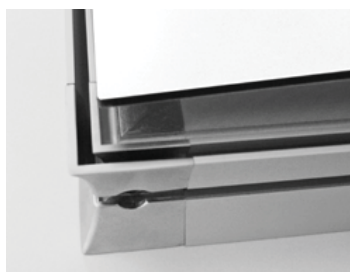
posizionare il pannello sulla cornice paneel in den rahmen legen place the panel on the frame
